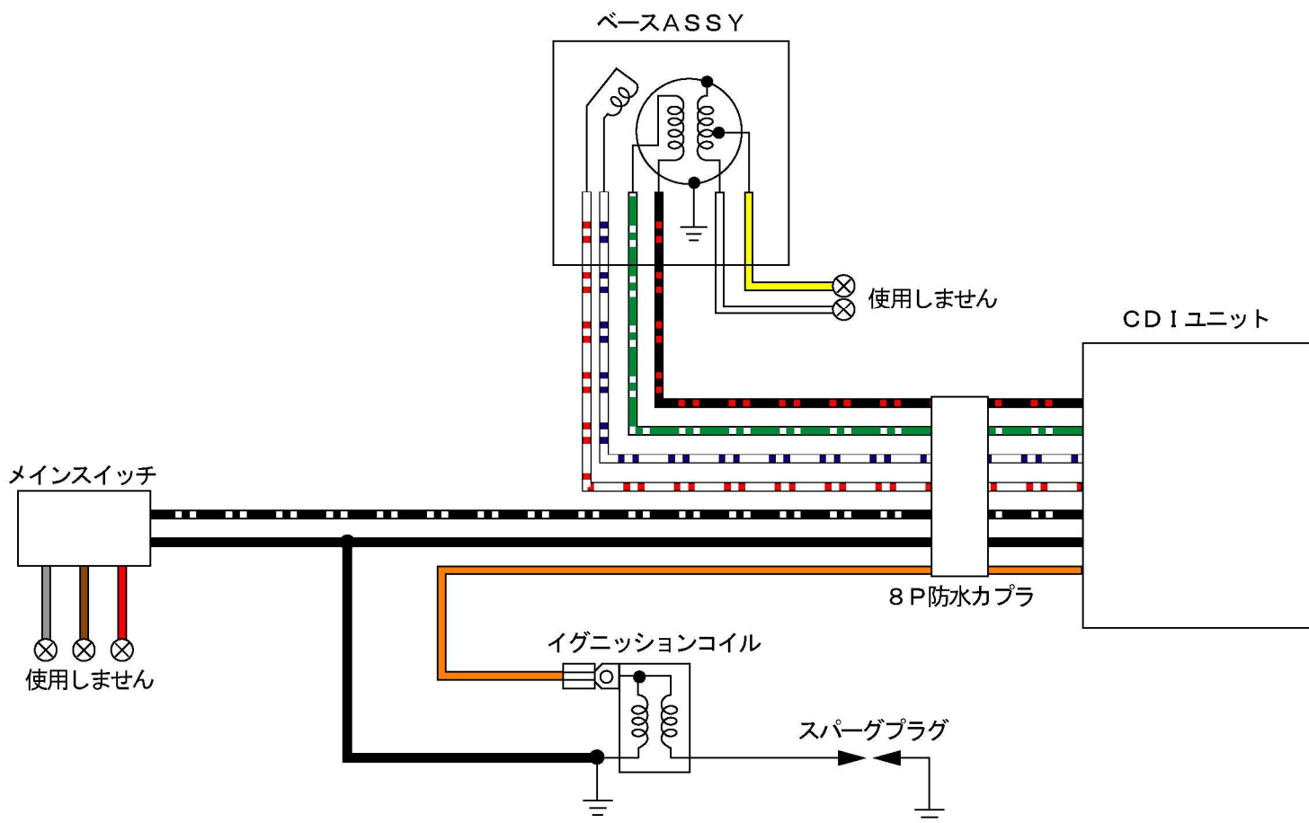
配線色一覧
